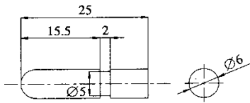
图 2 钉头
