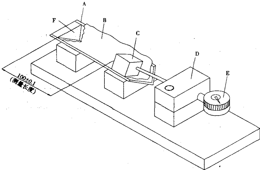
图 4 变形测定仪
