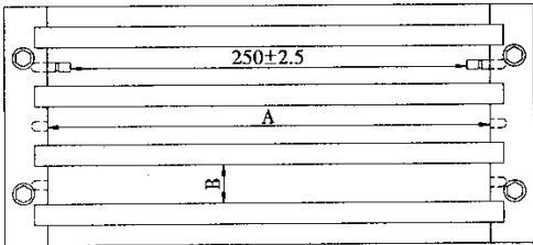
图 1 三联试模
